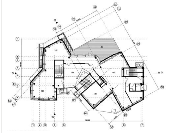
План 1-го этажа на отметке +0.000
