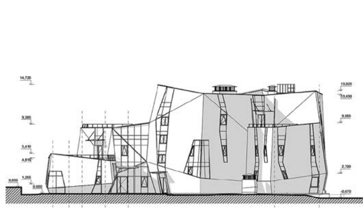
Фасад в осях 1-7
